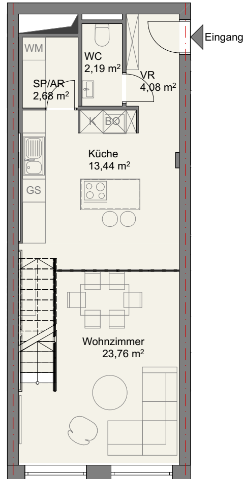
1.Obergeschoss
