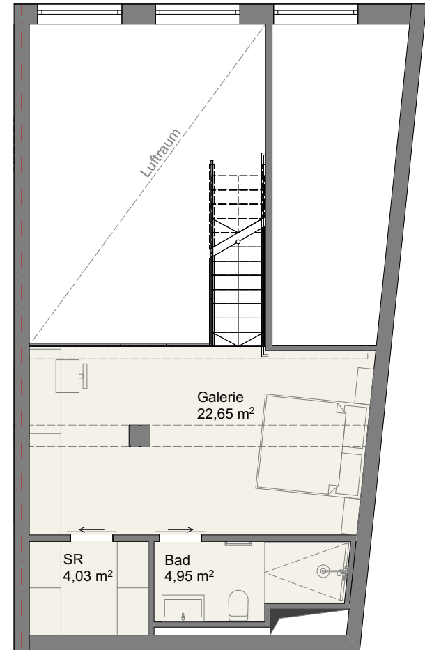
4.Obergeschoss/Galerie
